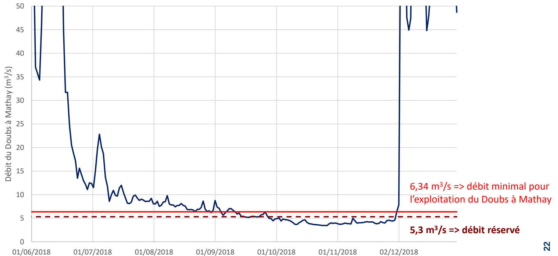
Débit du Doubs à Mathay pendant l'étiage de 2018
