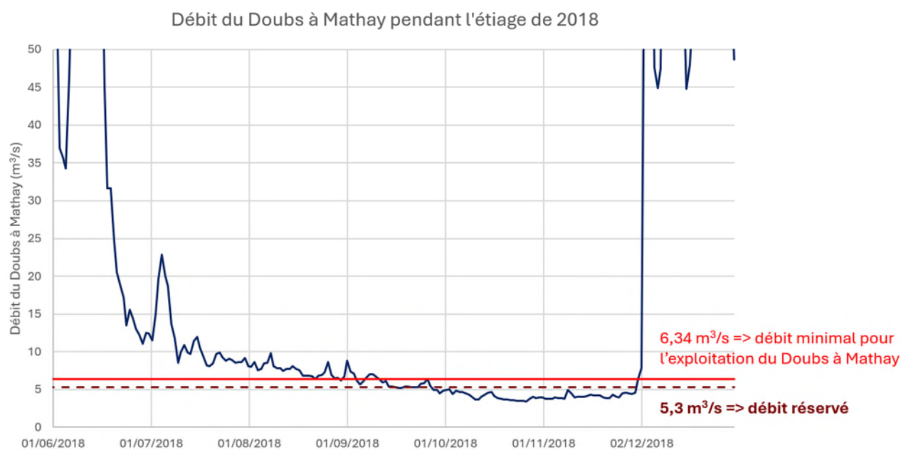
Figure 11 : Débit du Doubs à Mathay pendant l'étiage de 2018
